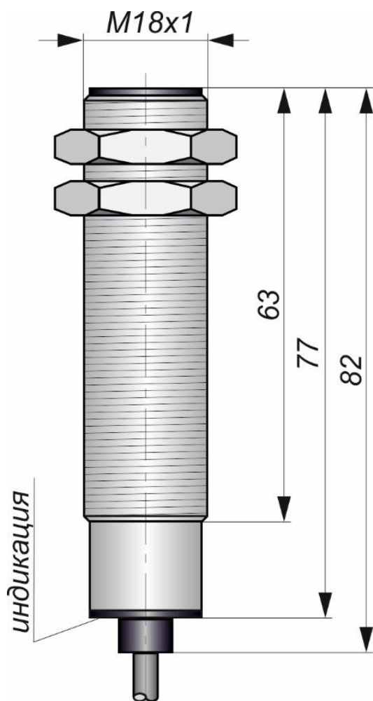
Габаритный чертеж
